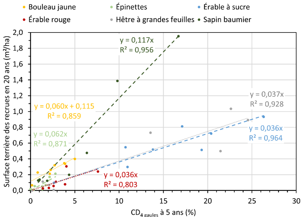
Figure A2.1. Relations entre la surface terrière des recrues observées 20 ans après la coupe de jardinage et le coefficient de distribution des gaules (CD 4_gaules ) estimé 5 ans après la coupe, pour 6 essences. Les lignes pointillées de différentes couleurs montrent la modélisation des observations. L'estimation des paramètres et le coefficient de détermination ( R^2 ) de chaque régression sont indiqués dans la couleur correspondante. Les pentes des équations correspondent aux facteurs de conversion du CD 4_gaules observé à 5 ans en surface terrière recrutée à 20 ans. L'ordonnée à l'origine est présentée seulement lorsqu'elle était significativement différente de 0 au seuil d'erreur \alpha = 0,05 .
