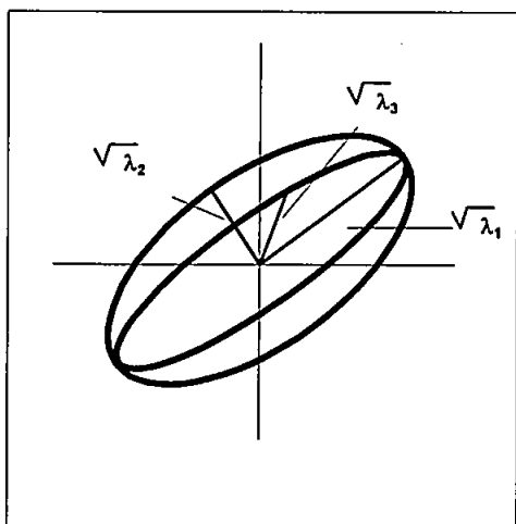
Figure 10. Ellipsoïde de variance-covariance; axes principaux : \sqrt{\lambda_1} , \sqrt{\lambda_2} et \sqrt{\lambda_3} .
