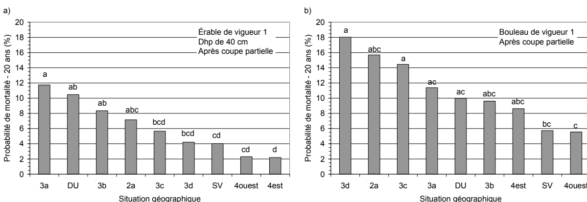
Figure 2.1. Probabilité de mortalité de l'érable à sucre (a) et du bouleau jaune (b) sur une période de 20 ans selon la situation géographique. Les lettres différentes sur les graphiques indiquent des différences significatives.
