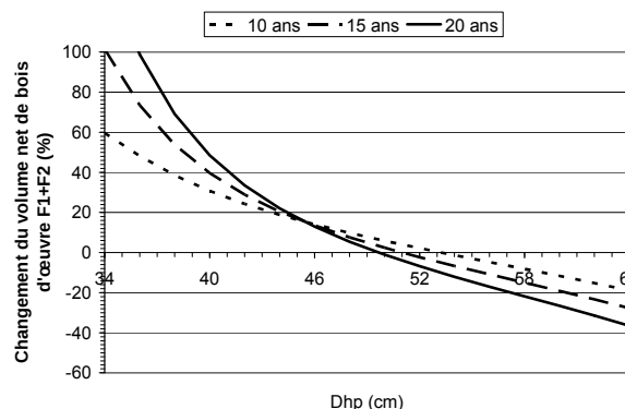
Figure 2.3 Exemples de changements du volume net de bois d'œuvre sur des périodes de 10, 15 et 20 ans pour l'érable à sucre dans la région écologique 3b (a) et pour le bouleau jaune dans la sapinière à bouleau jaune de l'ouest (b).
