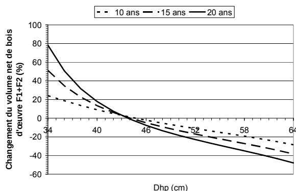
Figure 2.3 Exemples de changements du volume net de bois d'œuvre sur des périodes de 10, 15 et 20 ans pour l'érable à sucre dans la région écologique 3b (a) et pour le bouleau jaune dans la sapinière à bouleau jaune de l'ouest (b).
