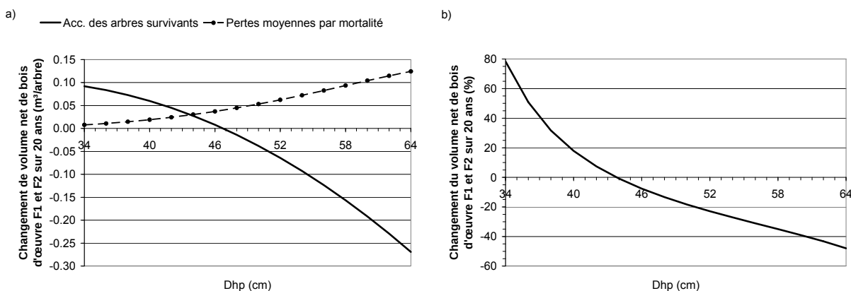
Figure 2.2. Observations de changement du volume net de bois d'œuvre de haute qualité (F1 et F2) sur une période de 20 ans chez l'érable à sucre dans la région écologique 3b. Les modèles d'accroissement des arbres survivants et des pertes par mortalité sont représentés dans la partie a), tandis que la somme de ces 2 modèles est représentée en valeurs relatives au volume initial dans la partie b).
